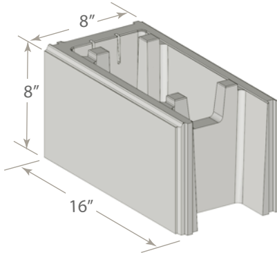
Tileco Mortarless Block End 8 x 8 x 16 ITEM #H088E
