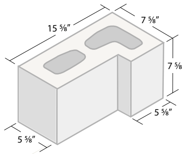
6 x 8 x 16 L-Return ITEM #068L
