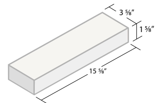
4 x 2 x 16 Cap ITEM #042
