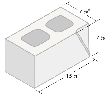
8 x 8 x 16 Shadowcaster Right*
