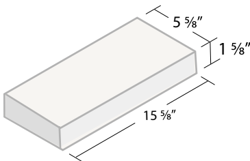
6 x 2 x 16 Cap ITEM #062
