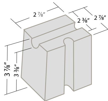
Dobies ITEM #DOBI5
