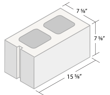
8 x 8 x 16 Jamb ITEM #088J
